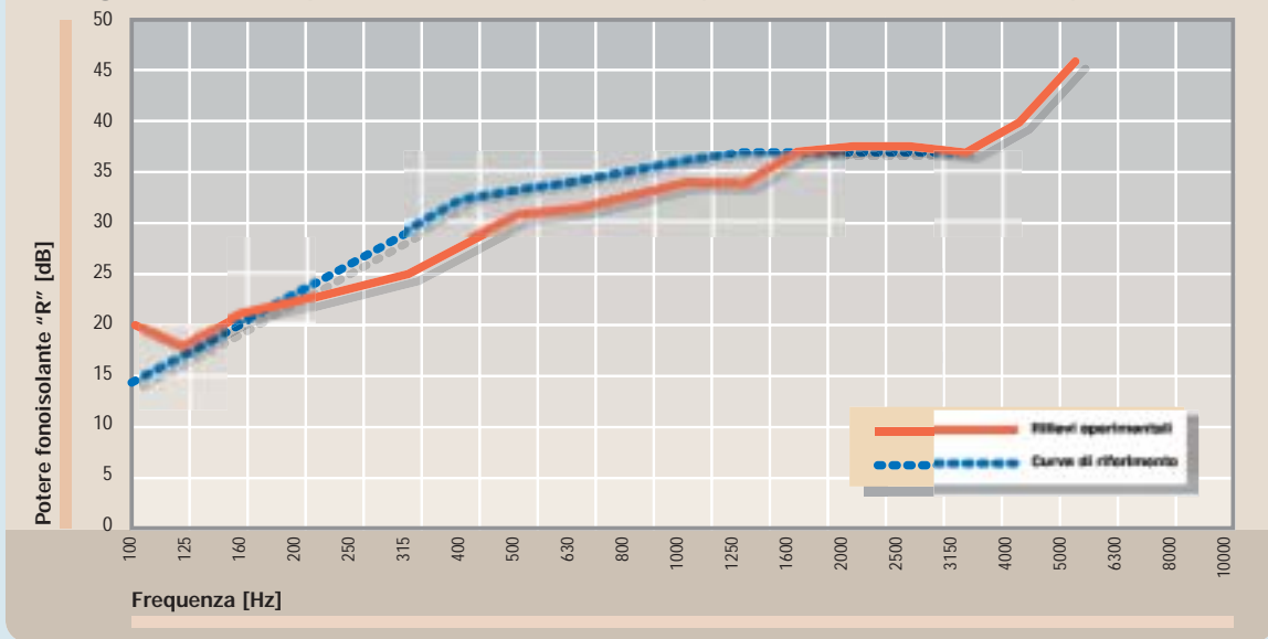
Diagramma del poterefonoisolante del pannello PENTA W.A. sp. 50 mm.
