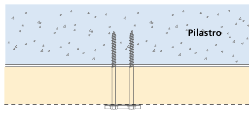
Vista in pianta
