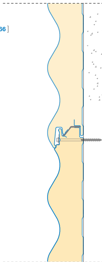
Vista in sezione
